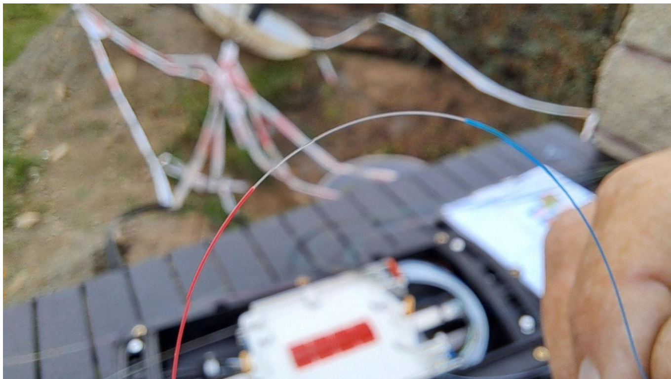
Foto č. 6 – komora v mlýnské ulici před RD č.p. 127 – svařené optické vlákno
