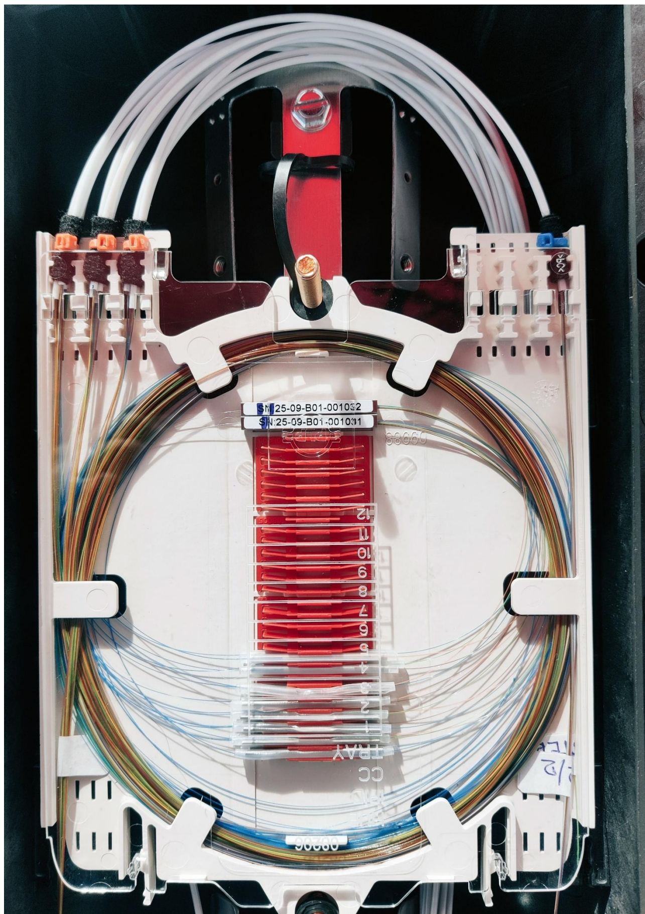
Foto č. 9 – uspořádání optických vláken v kazetě - komora KK2.4
